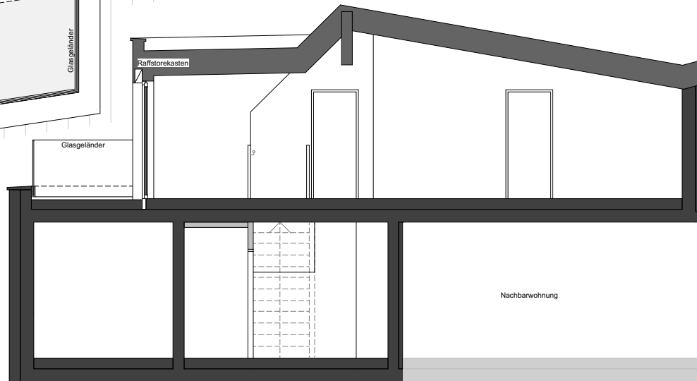
SCHNITT S-1
