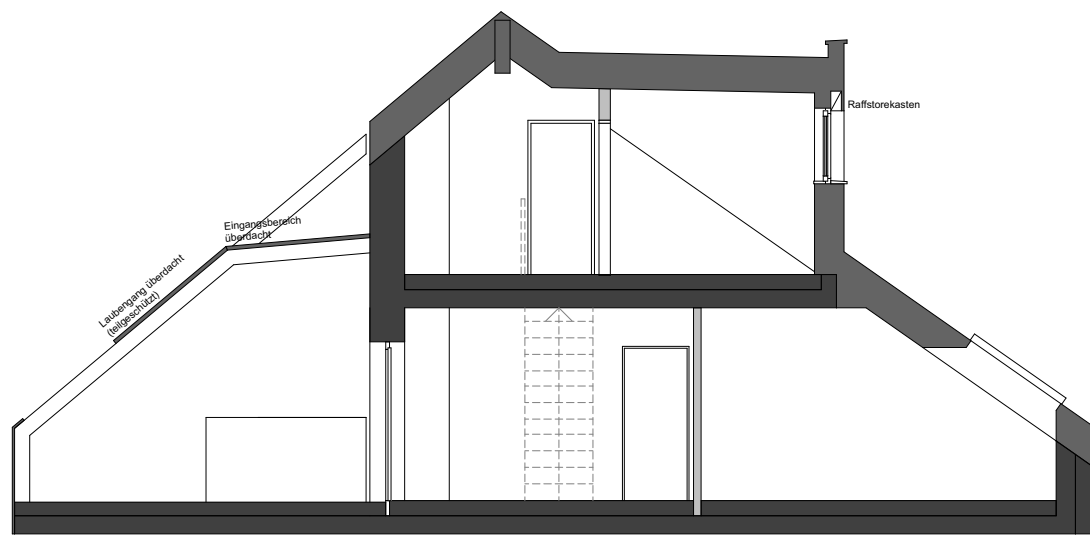
SCHNITT S-1
